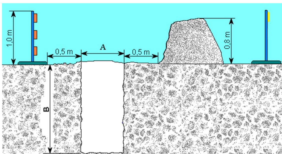
Munkaárok kialakítása, mérete 3.2.38 ábra
