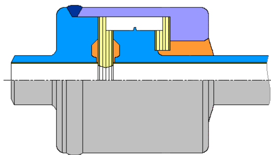
Elválasztó szigetelő közdarab 3.2.45 ábra
