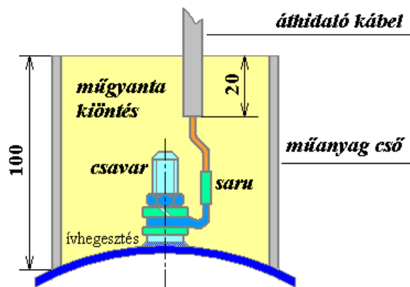
Fémes áthidalókötés 3.2.44 ábra
