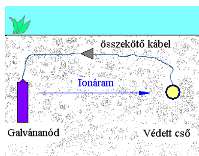
Galvánanódos védelem 3.2.48 ábra
