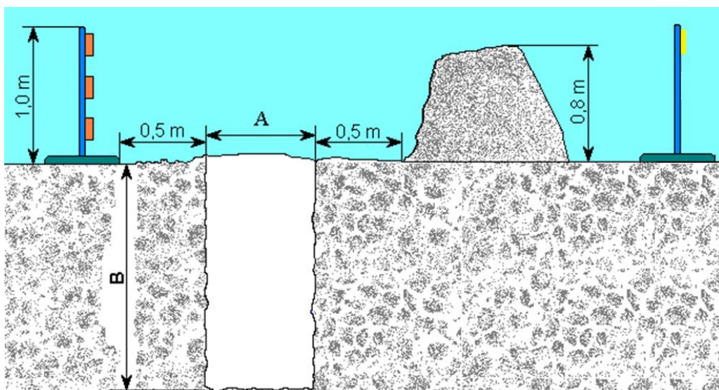
Munkaárok kialakítása, mérete 3.2.43 ábra
