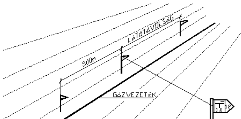
Jelzőoszlop beültetése egyenes csőszakaszon 3.2.59 ábra
