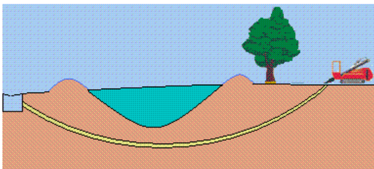
Irányított fúrás 3.2.42 ábra
