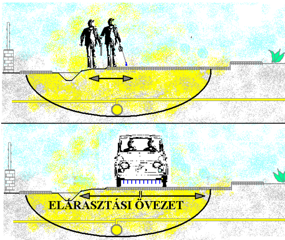
Tömörsegellenőrzés alkalmazhatósági tartománya 3.3.62 ábra
