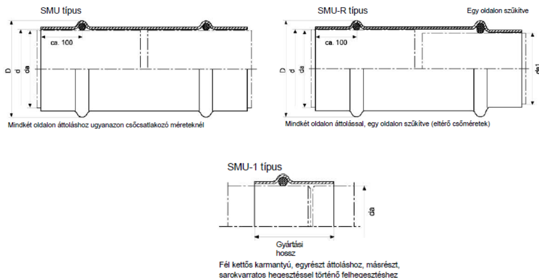
Áttoló karmantyú típusok 3.3.74 ábra
