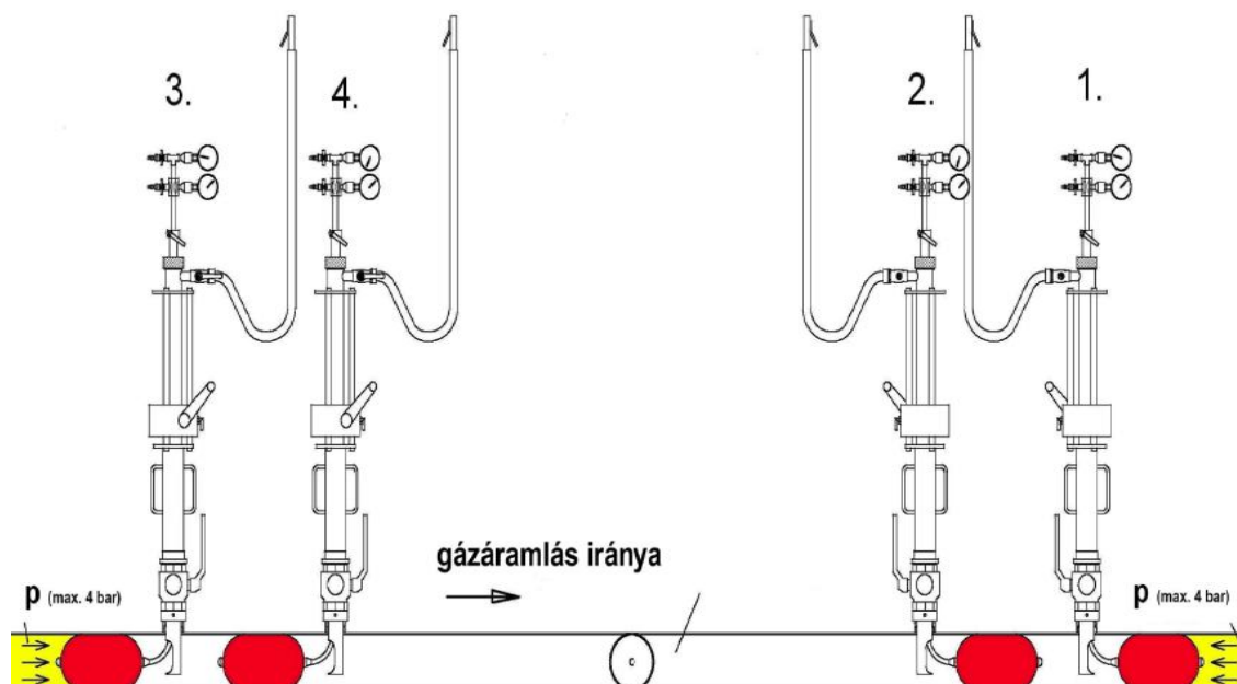
4 bar-os gépi ballonozó berendezéssel kiszakaszolt vezeték 3.3.73 ábra
