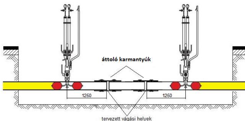
Gépi ballonozó berendezéssel kiszakaszolt vezeték 3.3.72 ábra
