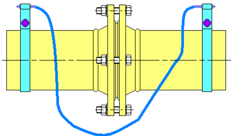
Ideiglenes, bilincses elektromos áthidaló 3.3.82 ábra
