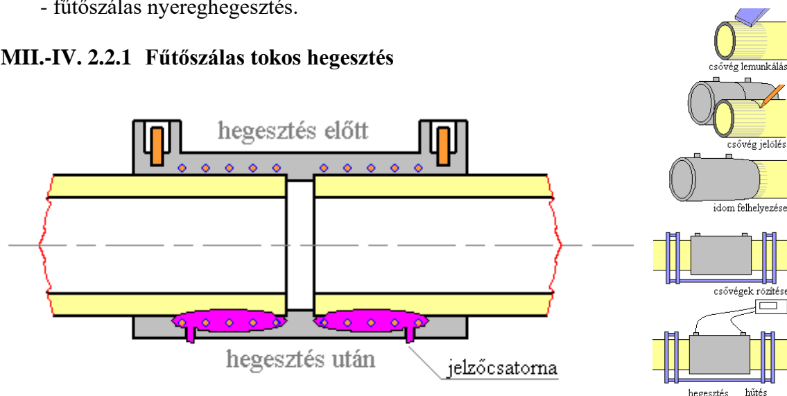
II.94 ábra Fűtőszálas tokos hegesztési varrat
