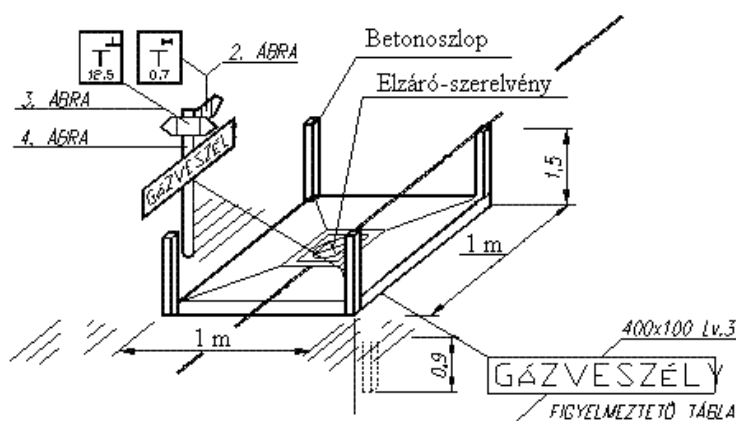
Külterületi szakaszoló elzáró védelme és jelölése 3.2.61 ábra
