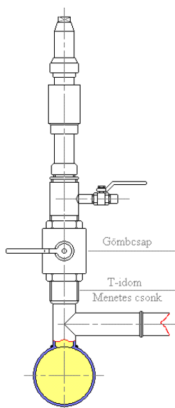
Acélcső nyomás alatti megfúró berendezés 3.3.79 ábra
