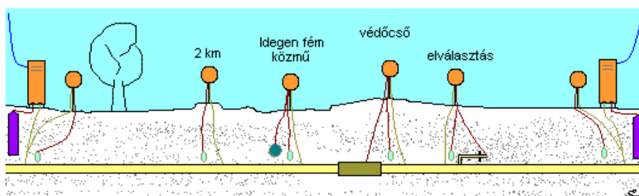
Katódállomások és potenciál-mérőhelyek 3.2.47 ábra
