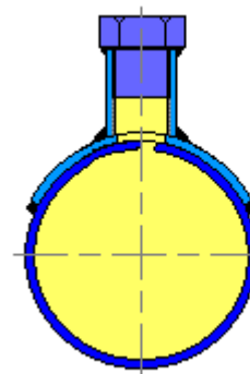
Acélkarmantyú 3.3.85 ábra
