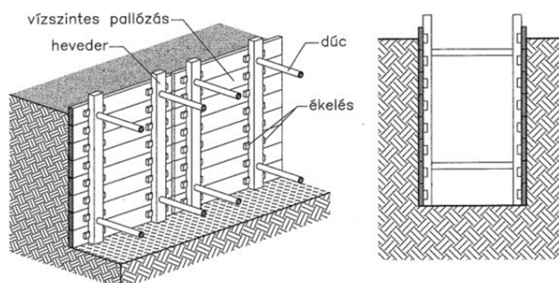
Vízszintes pallózású zárt dúcolás (Minta) 3.2.37 ábra
