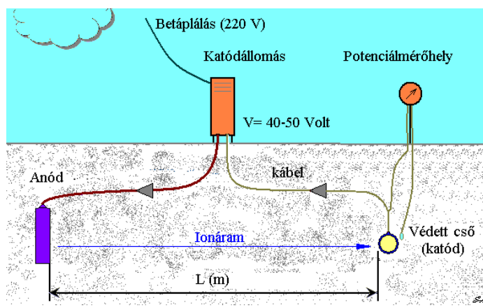
Külső áramforrással táplált katódos védelem 3.2.46 ábra
