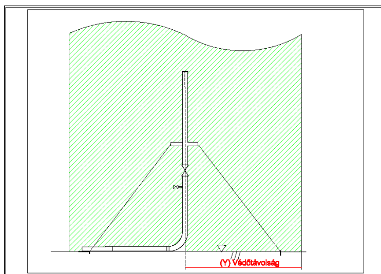
Védőtávolság kijelölésének módja 3.3.65 ábra
