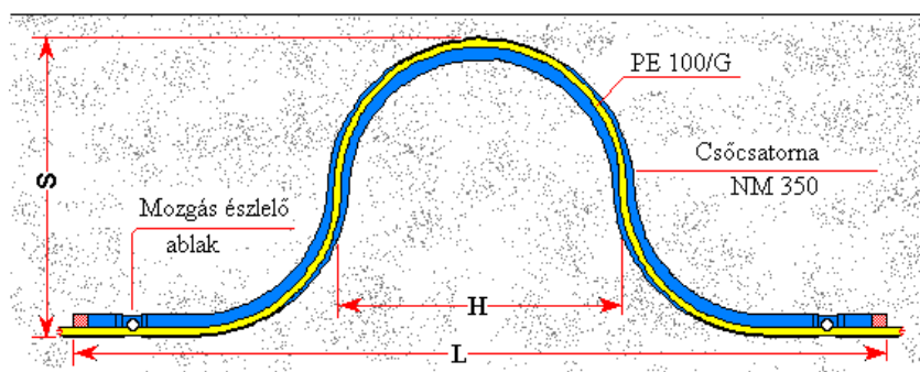
OMEGA – kompenzátor
