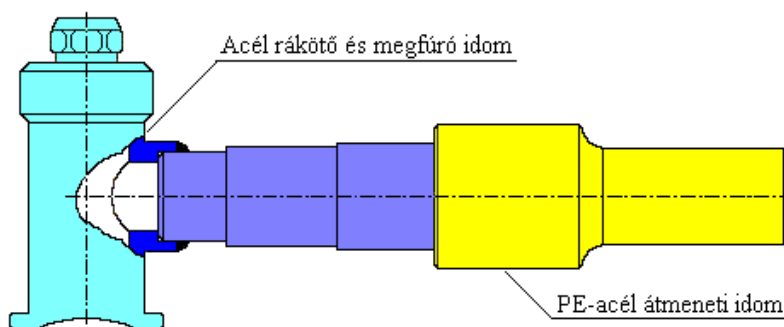
Acél megfúró idom PE-acél átmeneti idommal egybeépítve 3.1.32 ábra
